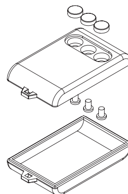
Eco Keyfobs (Serie 2597) 2957
